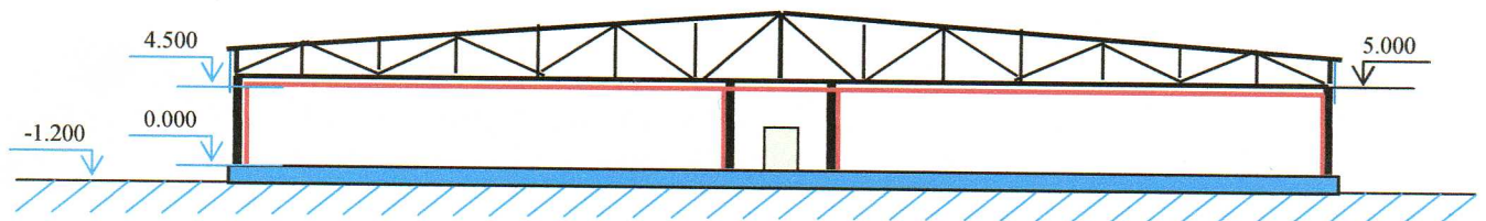
Разрез 1 – 1
